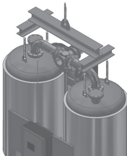
Kuljetus nosturilla
